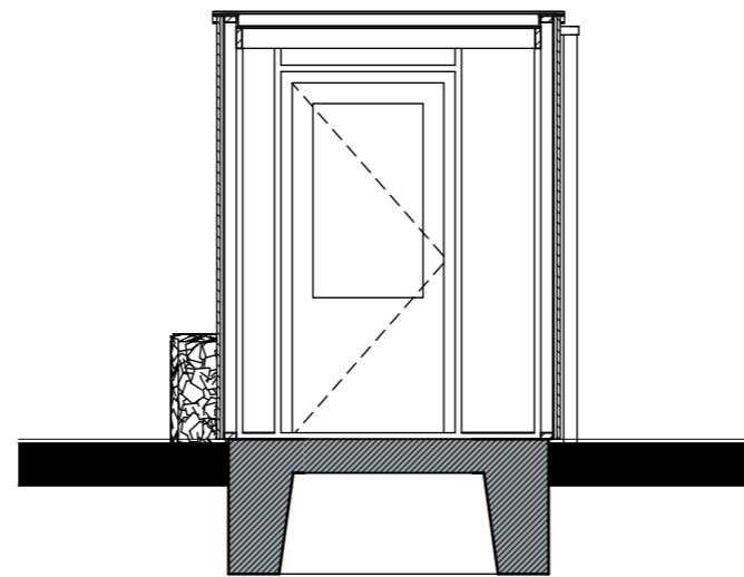
Doorsnede B-B
