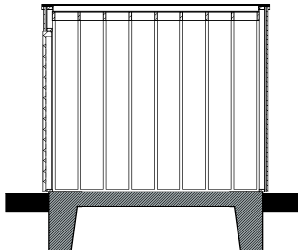
Doorsnede A-A
